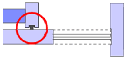
▲テープ付きモヘア断面
